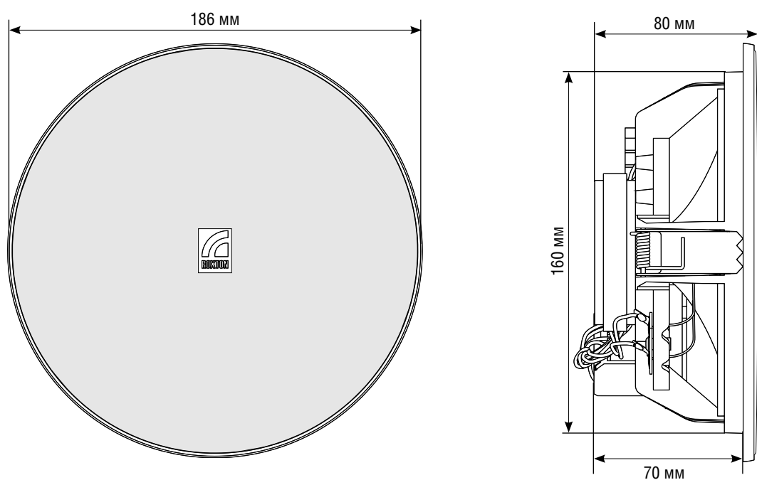
Рисунок А.1 Габаритные размеры ROXTON LF-06WT/BT
