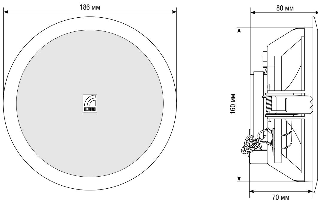
Рисунок А.1 Габаритные размеры ROXTON LF-06WT/BT
