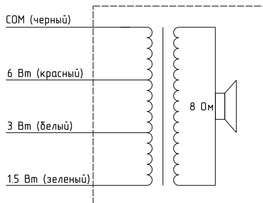
Рисунок 5.1 Принципиальная схема оповещателя
